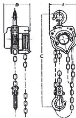
V-ACE手拉吊車
